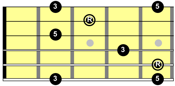
Pattern 1 Arpeggio
